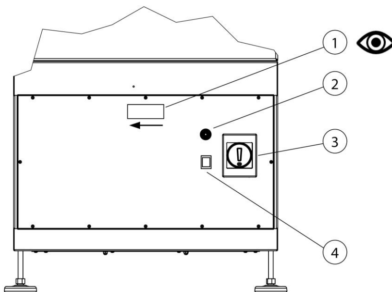
Sl. 5: Preverite smer vrtenja ventilatorja
