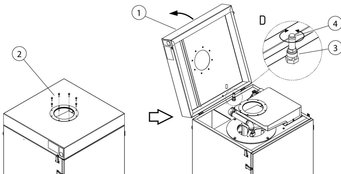
Sl. 12: Dostop do varnostnega ventila stisnjenega zraka
