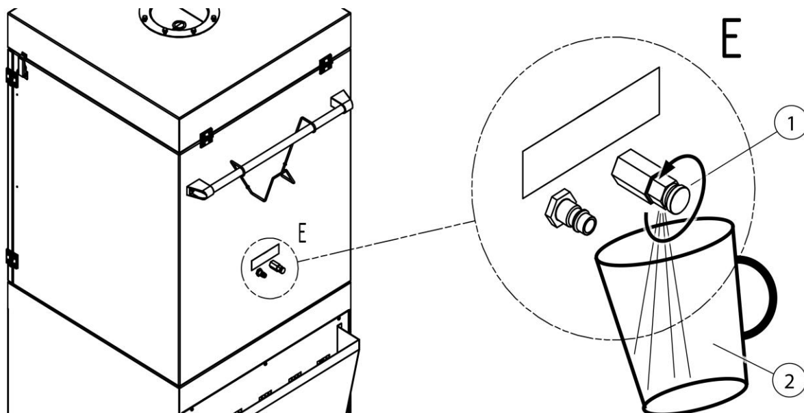
Sl. 8: Izpustite kondenzat
