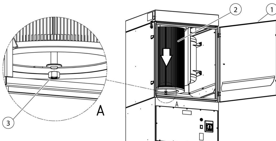
Sl. 9: Menjava filtra
